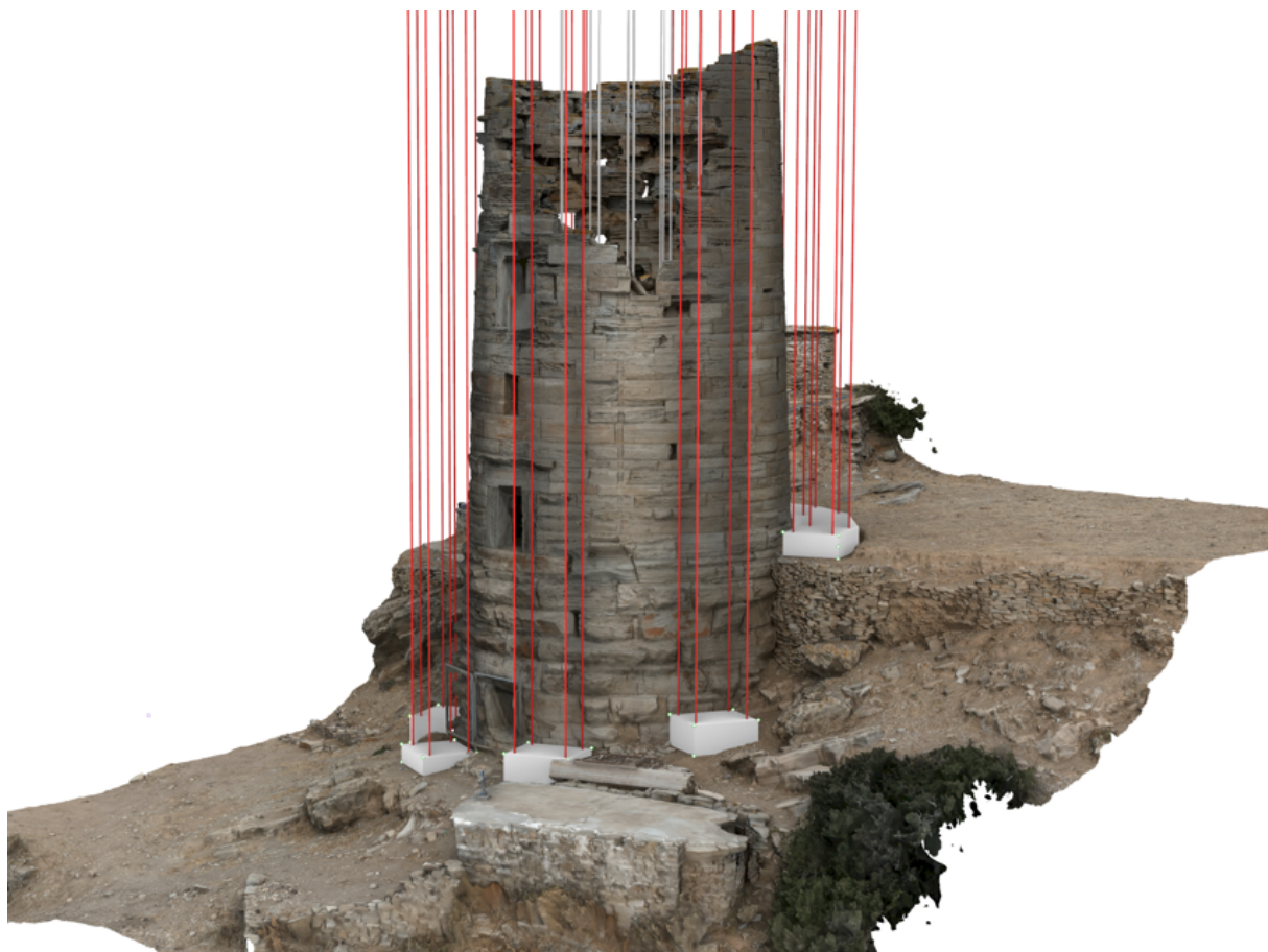
Εικόνα 2 Ο πύργος με τις βάσεις και τις θέσεις τοποθέτησης των εξωτερικών πύργων του ικρίωματος από νότιοανατολικά.
